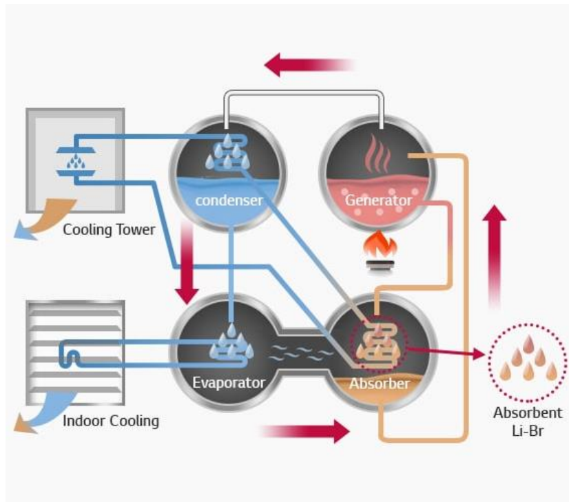
Schema de principiu a instalațiilor frigorifice prin absorbție echipate cu arzător https://www.lg.com/global/images/global-directfiredabsorptionchiller-pdp-1-d.jpg
