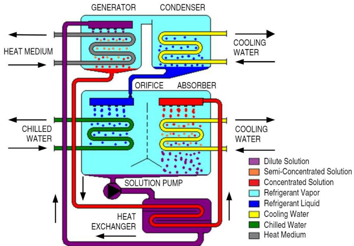
Schema de principiu a unui chiller prin absorbție, cu LiBr – apă http://www.yazakienergy.com
