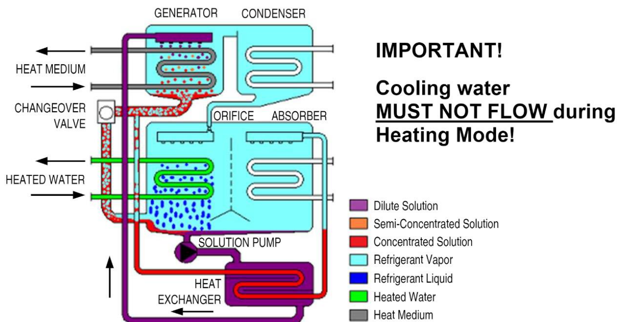
Schema de principiu a unui chiller prin absorbție, cu LiBr – apă (în regim de încălzire) http://www.yazakienergy.com
